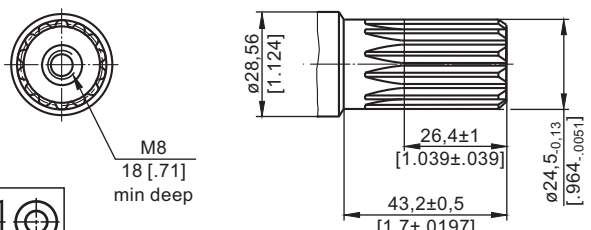
SA - splined, B25x22xH9 DIN 5482 Max. Torque 40 daNm [3540 lb-in]
